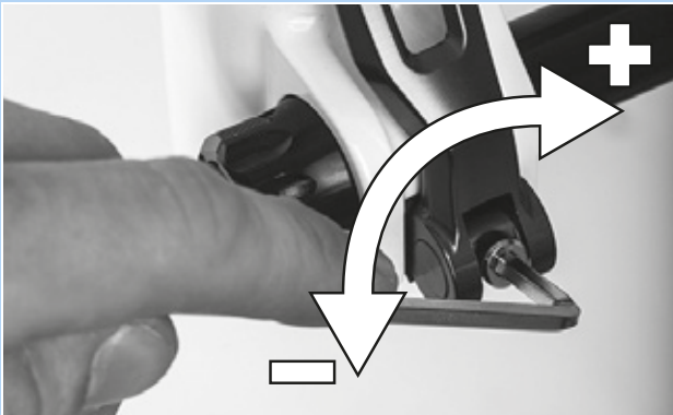
Afbeelding 146: Spankracht van de snelspanner afstellen
