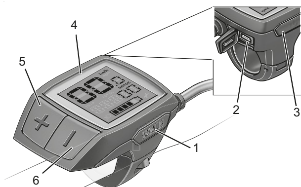
Afbeelding 110: Opbouw BOSCH Purion boordcomputer
