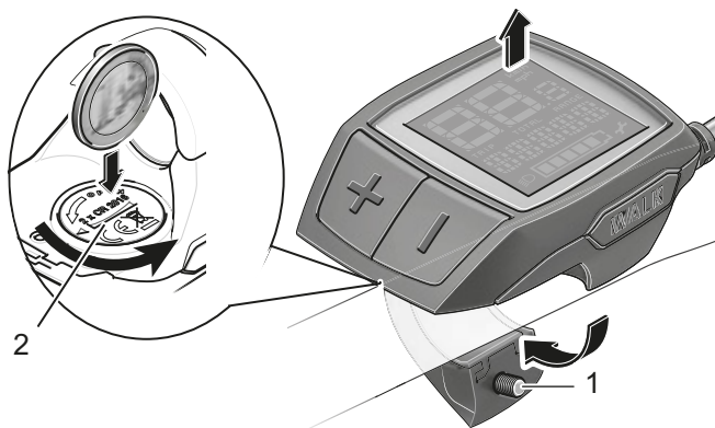
Afbeelding 124: Boordcomputer met bevestigingsschroef (1) en deksel (2) van het batterijcompartiment
