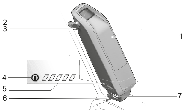
Afbeelding 30: Detail frame-accu
